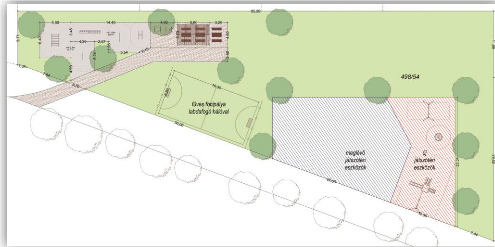
A tervezett játszóterébővítés és a kondipark helyszínrajza A Szent László lakóparkban
