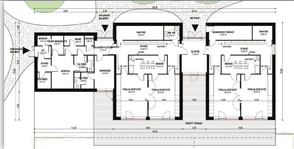
Családi bölcsőde vázlattevé, földszinti alaprajz
