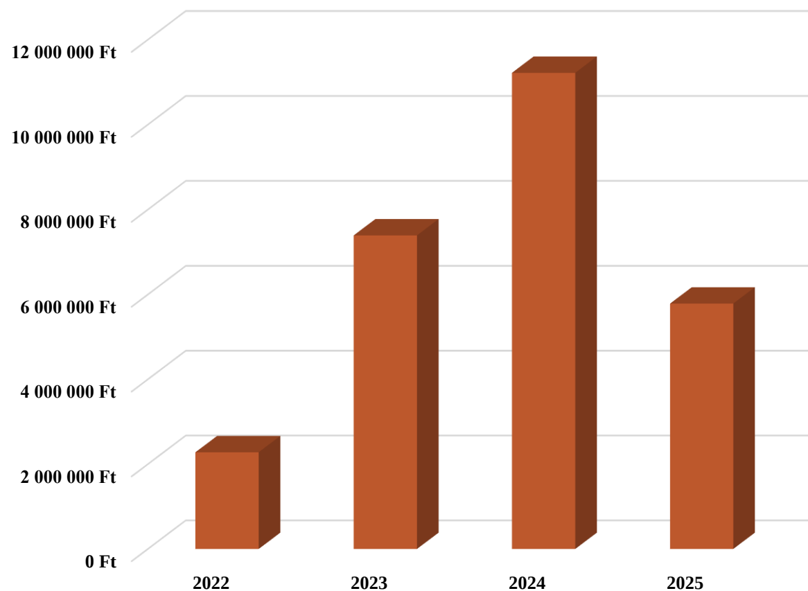
Adómérséklés alakulása
