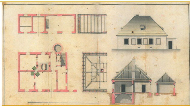
Az 1793-1794-ben felépült plébánia tervrajza (részlet)
